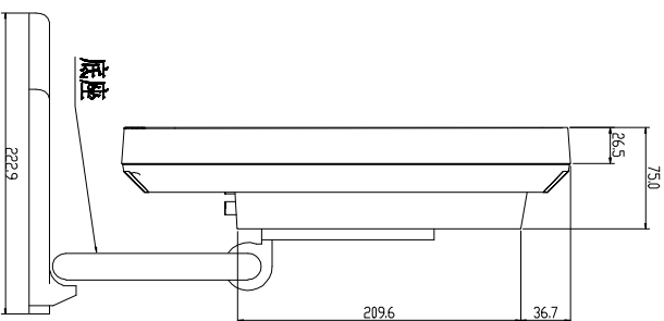
右侧视图
