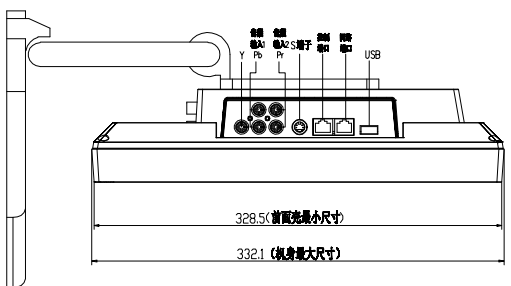
左侧视图
