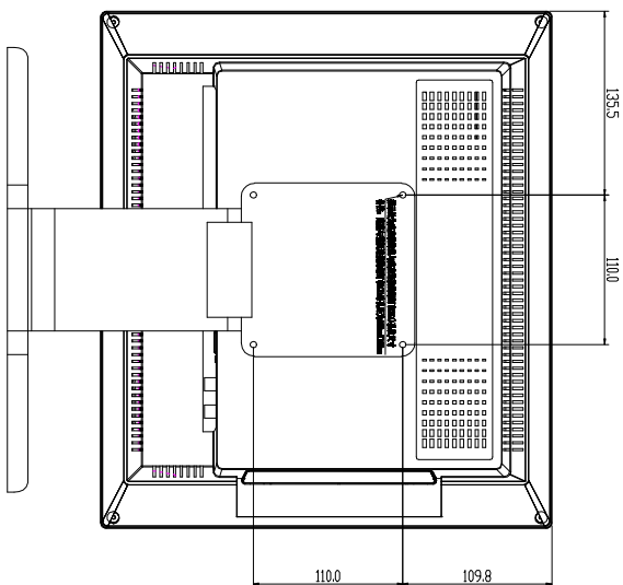
后视图
