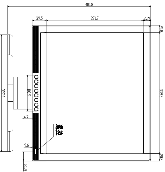
前视图
